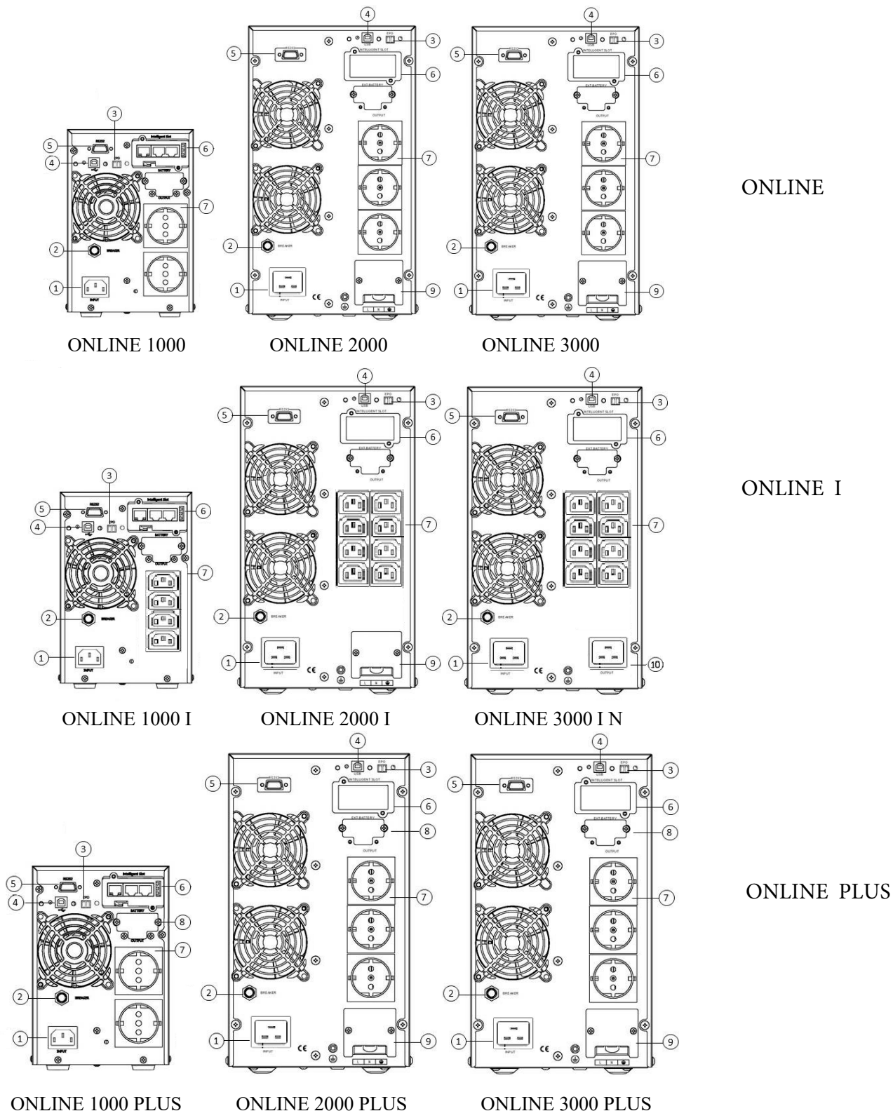
Рис.2 Схемы задних панелей ИБП
