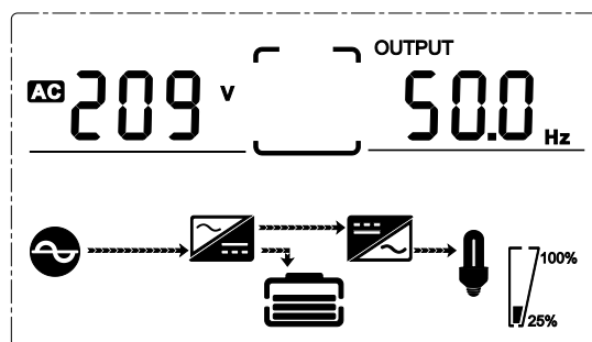
(3) Выходное напряжение
